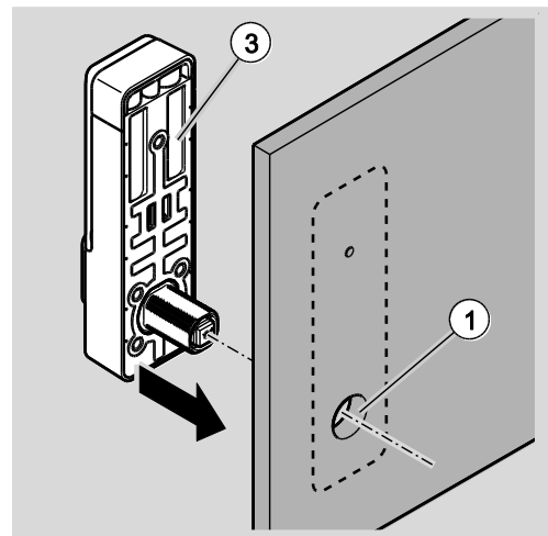
Abb. 10: Möbelverschluss durch die Einbaulochung schieben
