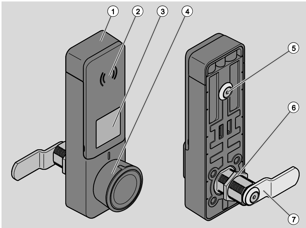
Abb. 4: Möbelverschluss mit rundem Drehknopf
