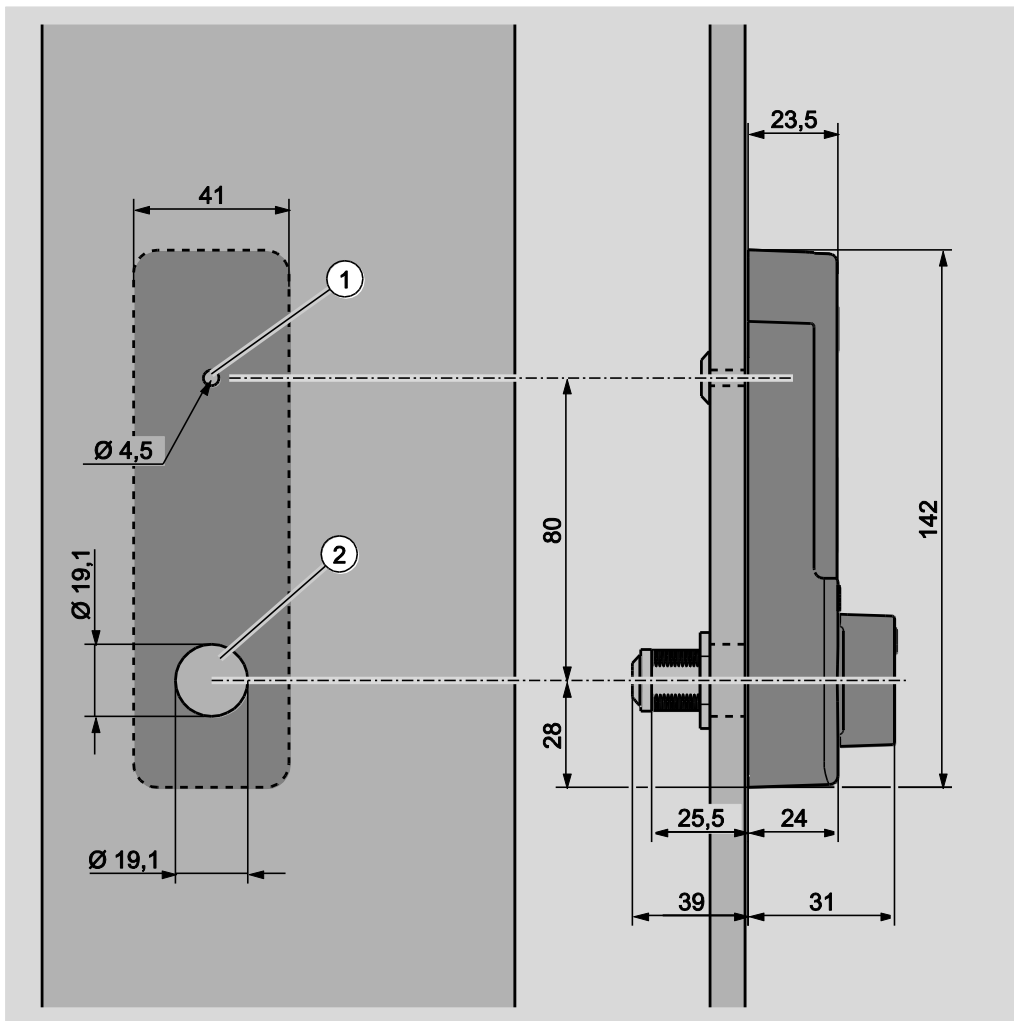
Abb. 7: Holztür vorbereiten
