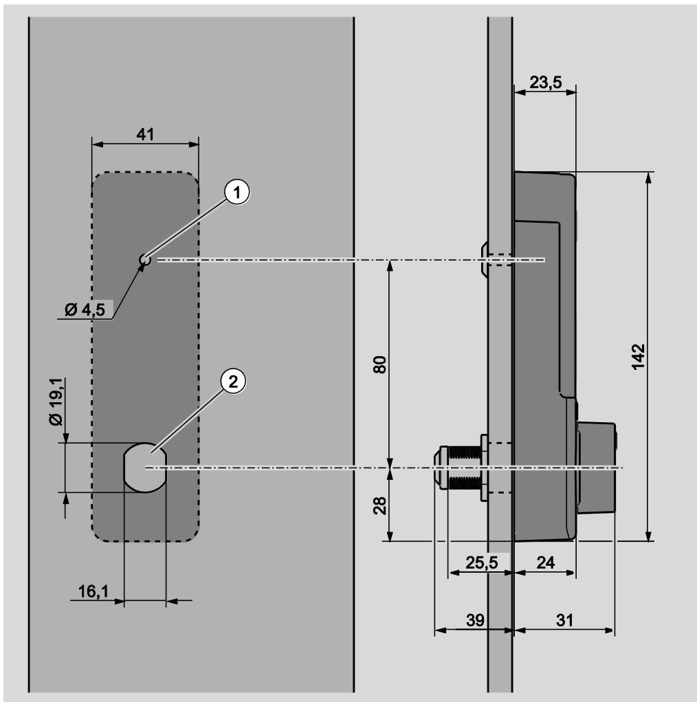
Abb. 8: Metaltür vorbereiten
