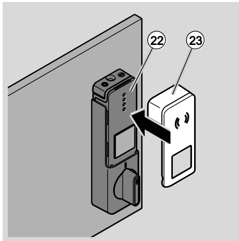
Abb. 21: Abdeckung am Möbelverschluss aufklipsen
