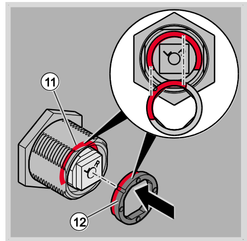
Abb. 14: Einbaulage des Einstellrings
