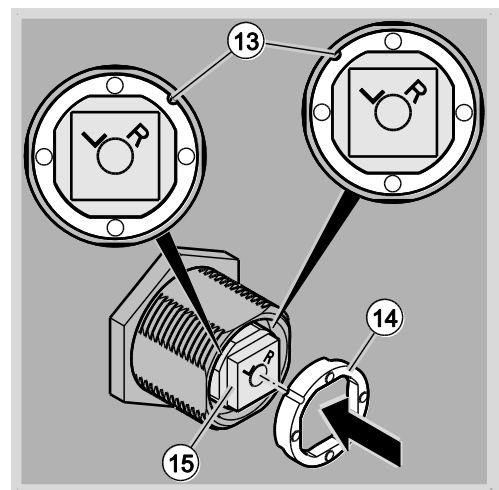
Abb. 15: Hebelposition festlegen
