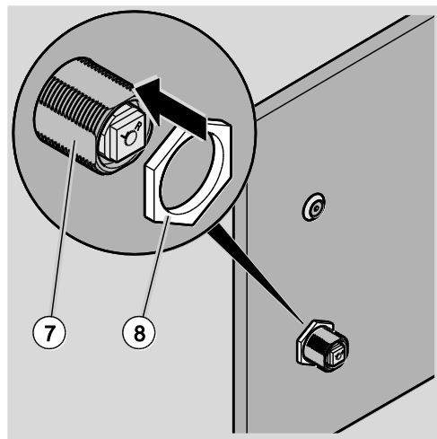
Abb. 12: Sechskantmutter aufsetzen
