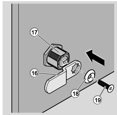
Abb. 18: Hebel montieren
