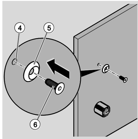
Abb. 11: Schraube einsetzen
