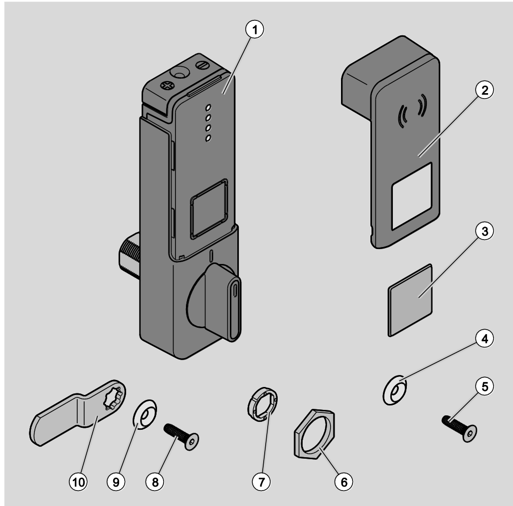
Abb. 1: Möbelverschluss mit schmalem Drehknauf
