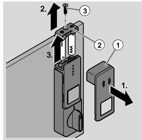
Abb. 27: Batterien wechseln
