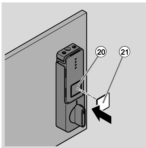
Abb. 20: Logoplatte anbringen
